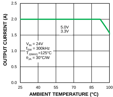
24V Input Thermal Derating MIC28512-1
